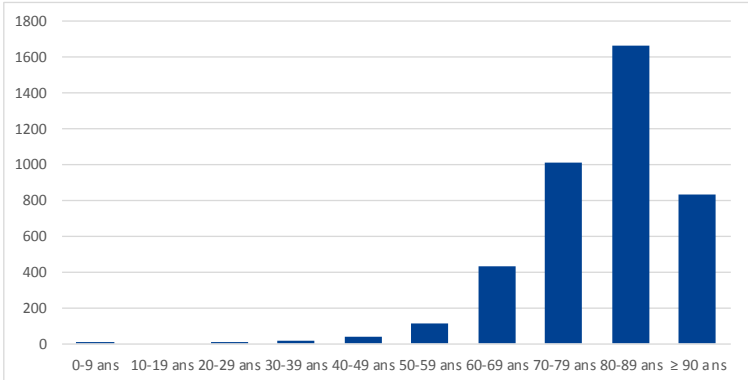
Figure 19. Distribution par classe d'âge des personnes décédées de Covid-19 par semaine depuis le 1er mars 2020. Grand Est
